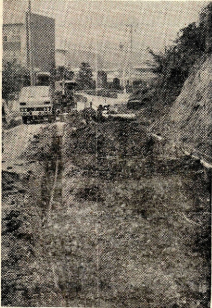
▲市道深川中学校西線上水道 給水管布設工事
