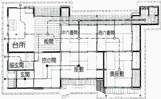
▲三隅山荘平面図
