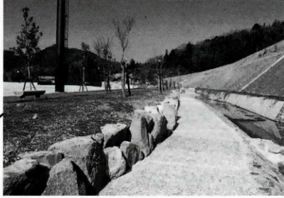
親水歩道（石置） 117m
