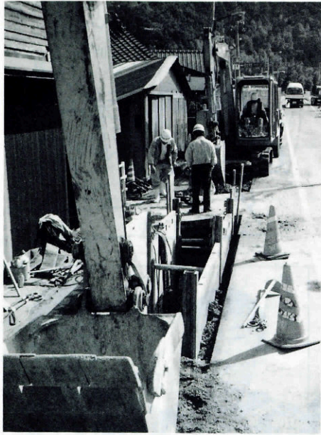
▲農業集落排水事業の管路布設（平成11年度には町の水洗化率94%の予定）
