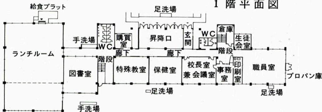
1 階平面図
